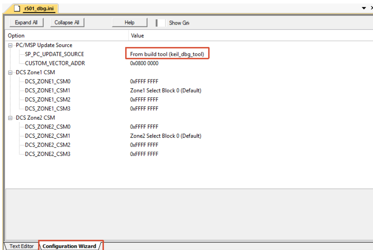
图 2 Configuration Wizard 配置界面
