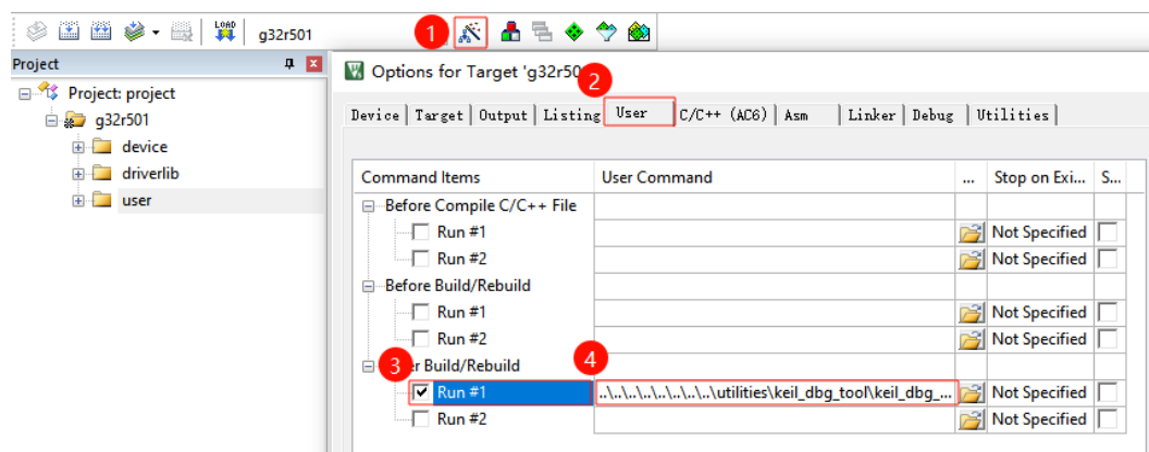
图 1 如何添加自定义的构建后步骤
